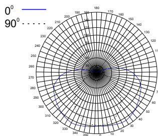
ЛПП-07В-1x36
