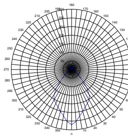
ГСП-19В-700-211
