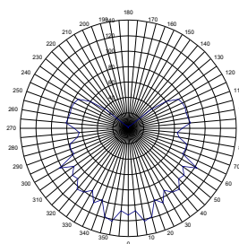
НСП-21ВEx-200-111
